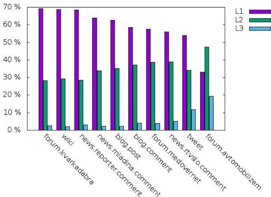
Slika 4: L-standardnost podkorpusov.
